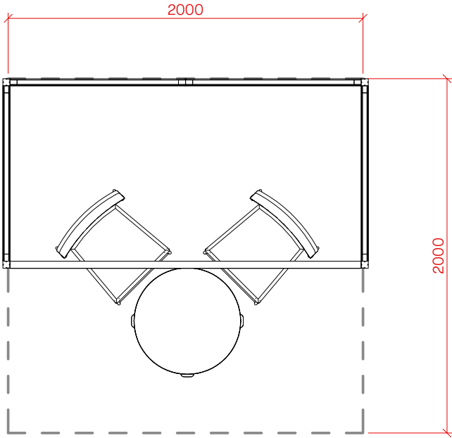
1 Plan View A03 1 : 30
