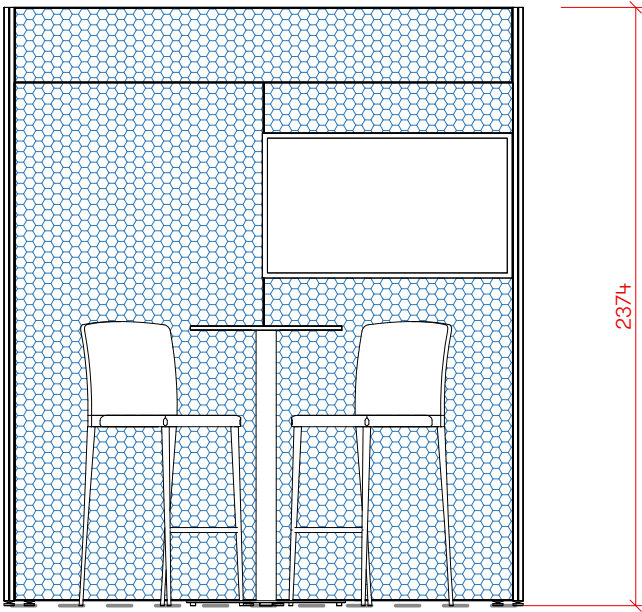
2 Elevation - Front A03 1 : 30
